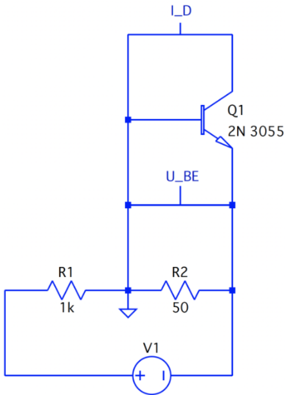
Abb. 4: Schaltskizze zur Bestimmung der Boltzmannkonstante mit einem 2N 3055 npn-Leistungstransistor [1]
