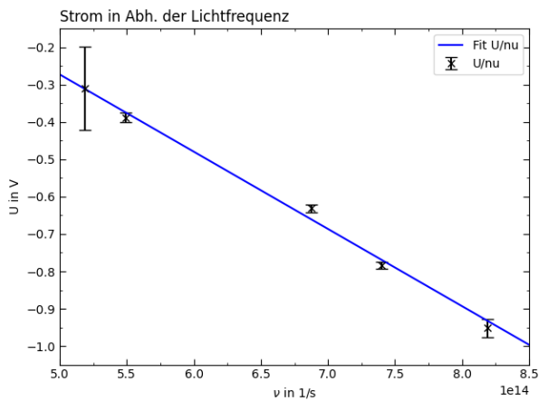
Abb. 3: Kniespannung der Photodiode in Abhängigkeit der Lichtfrequenz
